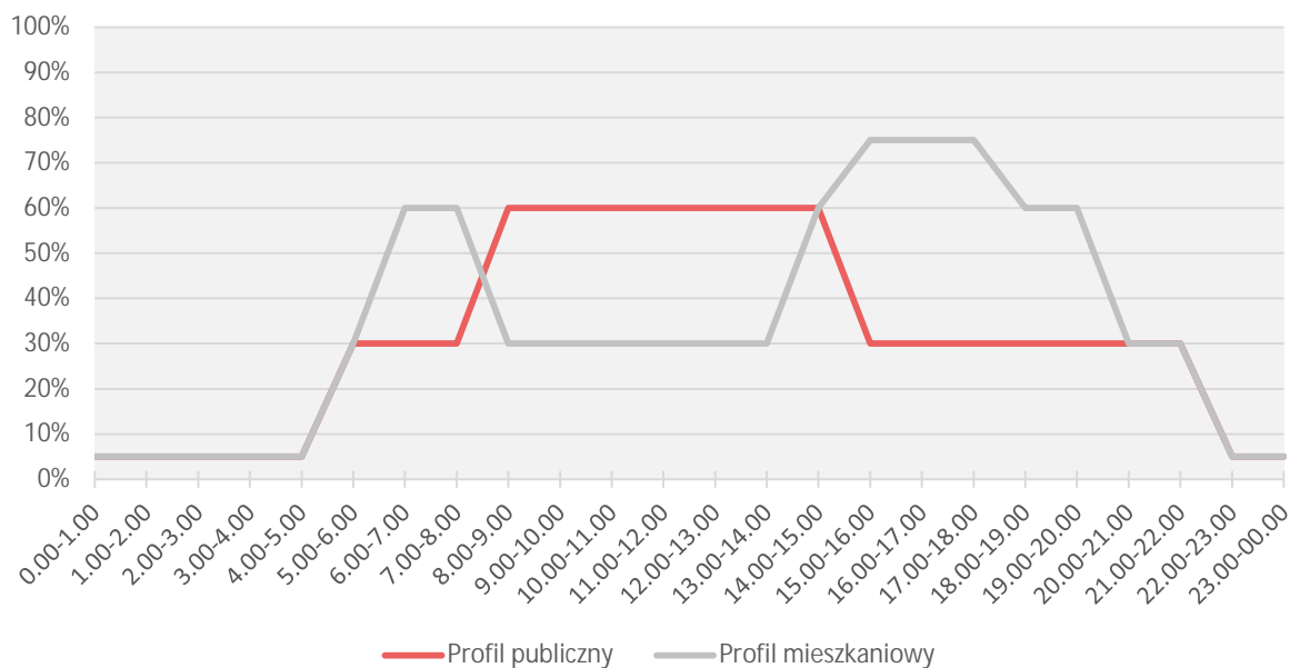
Rysunek 18: Charakterystyka dobowa wykorzystania stacji ładowania
